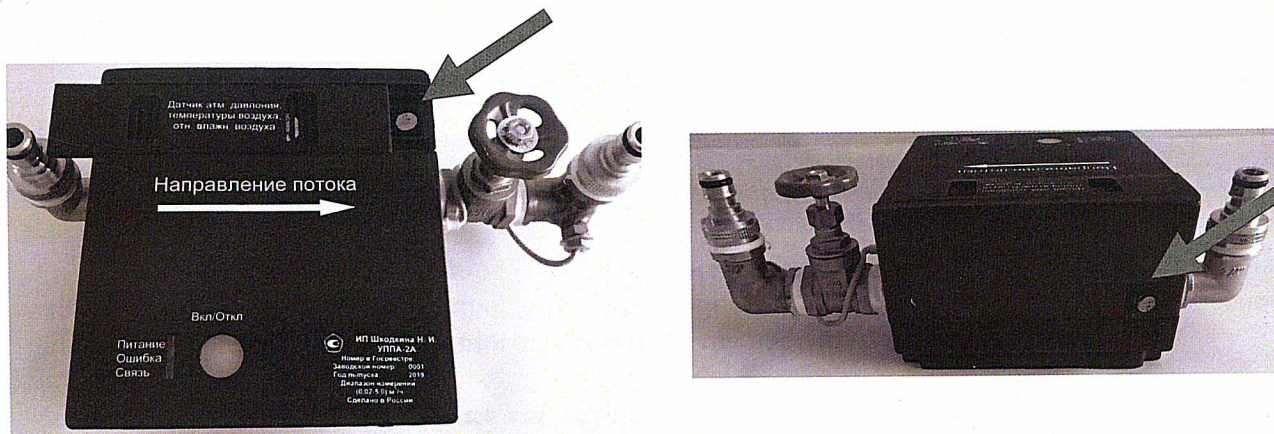
Рисунок 3 – Места нанесения знака поверки на установки модификации УППА-2-А и УППА-3-А
